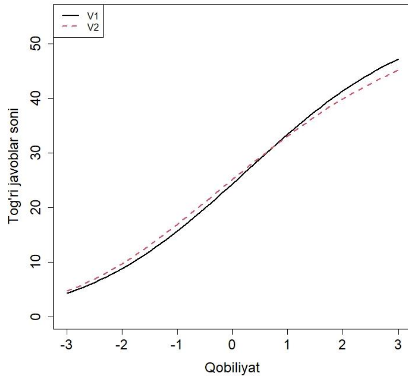
Test xarakteristikasi chiziqlari
